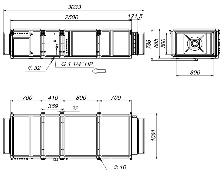
Левое исполнение
